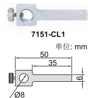
杠杆表支架(选配)
